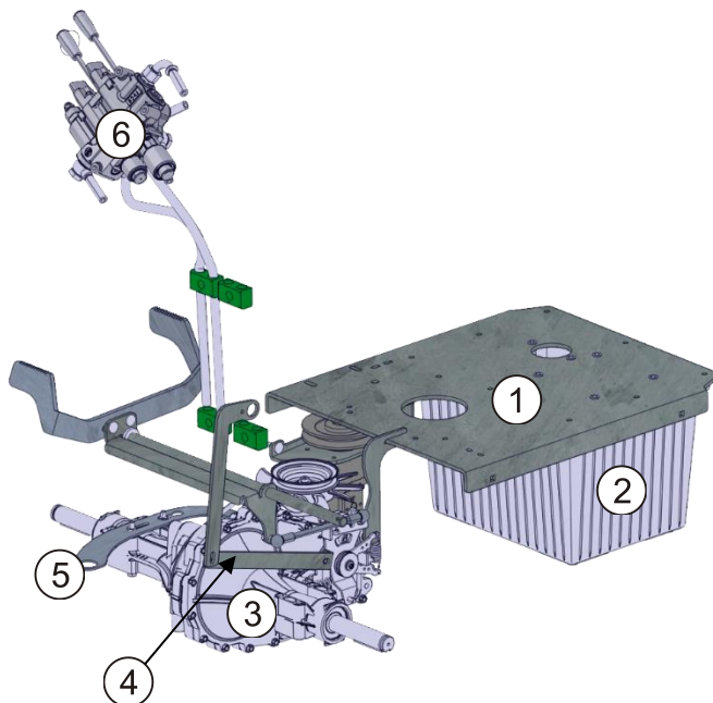
Abb. 30 - Antriebseinheit
