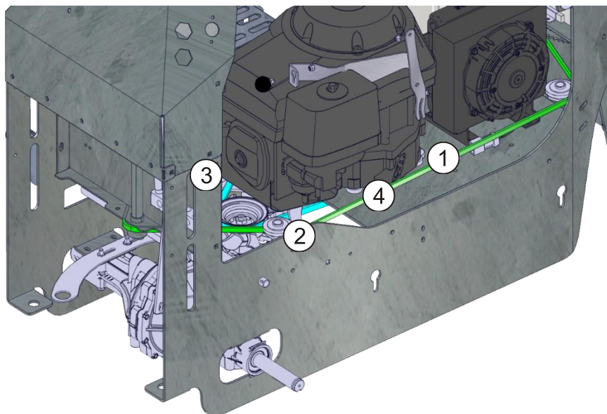
Abb. 27 - Riemen
