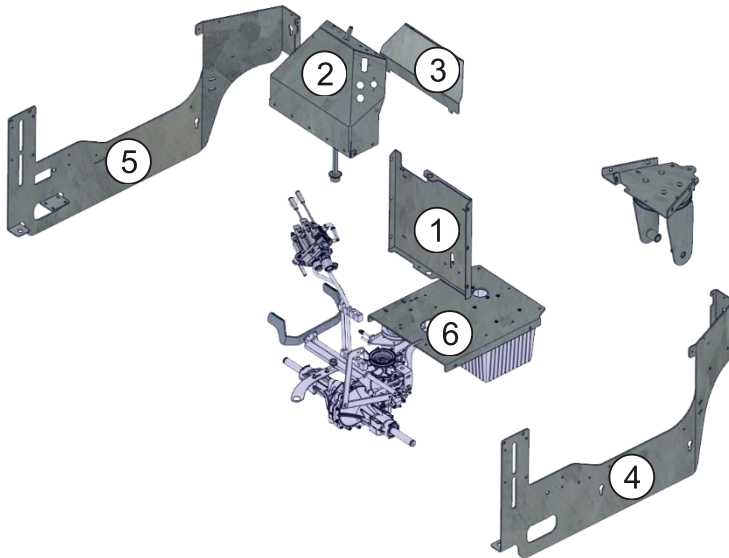
Abb. 29 - Gehäuse
